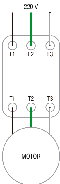
Línea Trifásica
