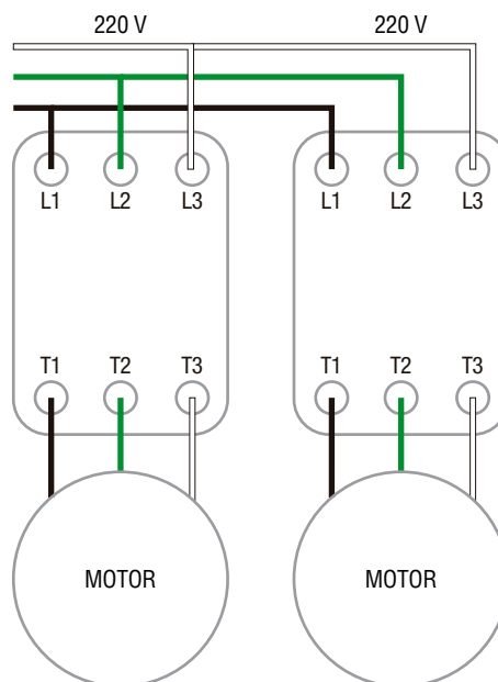
Línea Trifásica con dos motores
