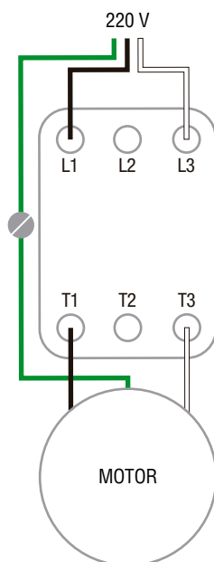
Línea Bifásica
